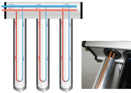
Princip för u-pipe solfångare
